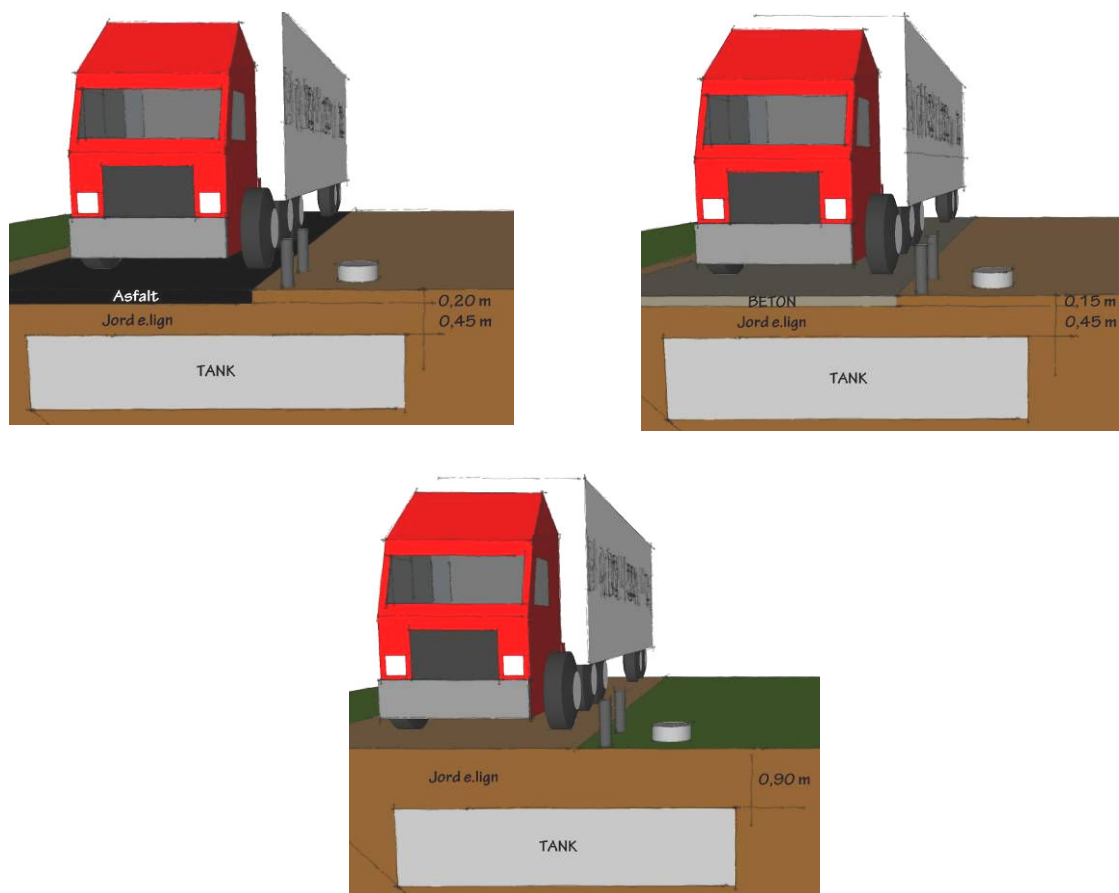
Figur 16: Illustration af forskellige belægninger, herunder tykkelse til beskyttelse af tanken mod trafiklast.
