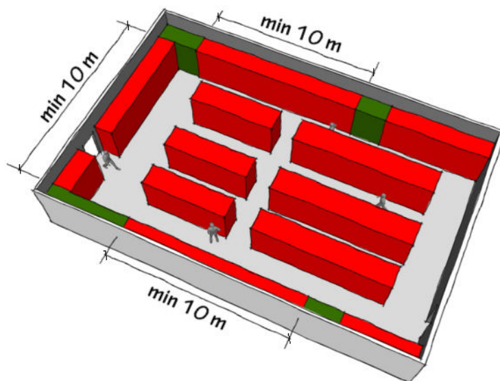
Figur 2: Indbyrdes placering af gasser i forhold til brandfarlige væsker i butikker uden brug af brandskabe.
