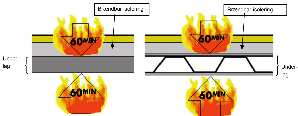
Figur 32: Brændbar isolering i tag på underlag af EI 60 A2-s1,d0.
