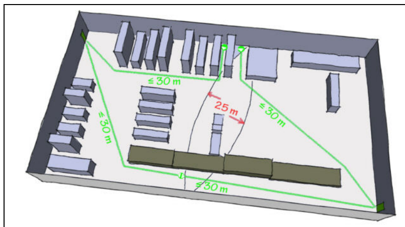
Figur 31: Indretning hvor både 25 og 30 m reglen er opfyldt.
