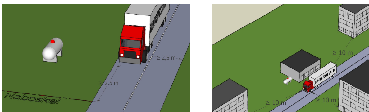
Figur 33: Illustration af afstandskrav i forhold til holdeplads.
