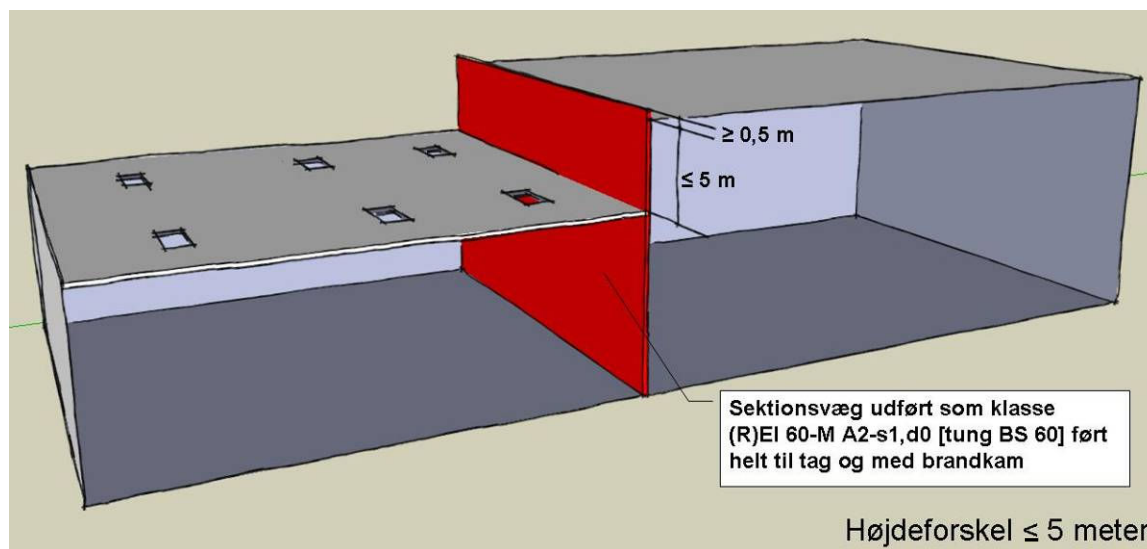
Figur 25: Sikring mod høj-lav brandsmitte, hvor den højere bygnings tag er mindre end eller lig med 5 m over den lavere bygnings tag. Løsning med brandkam.
