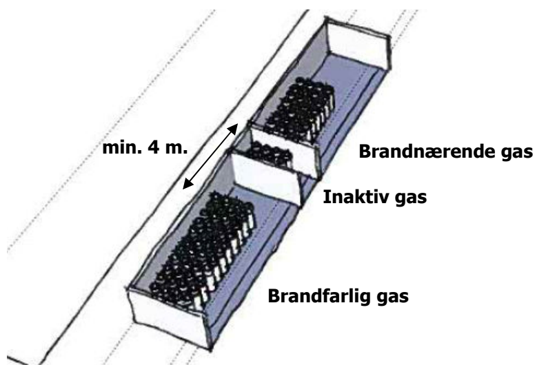
Figur 6: Eksempel på udnyttelse af det min. 4 m mellemrum der skal være mellem brandnærende og brandfarlige gasser.
