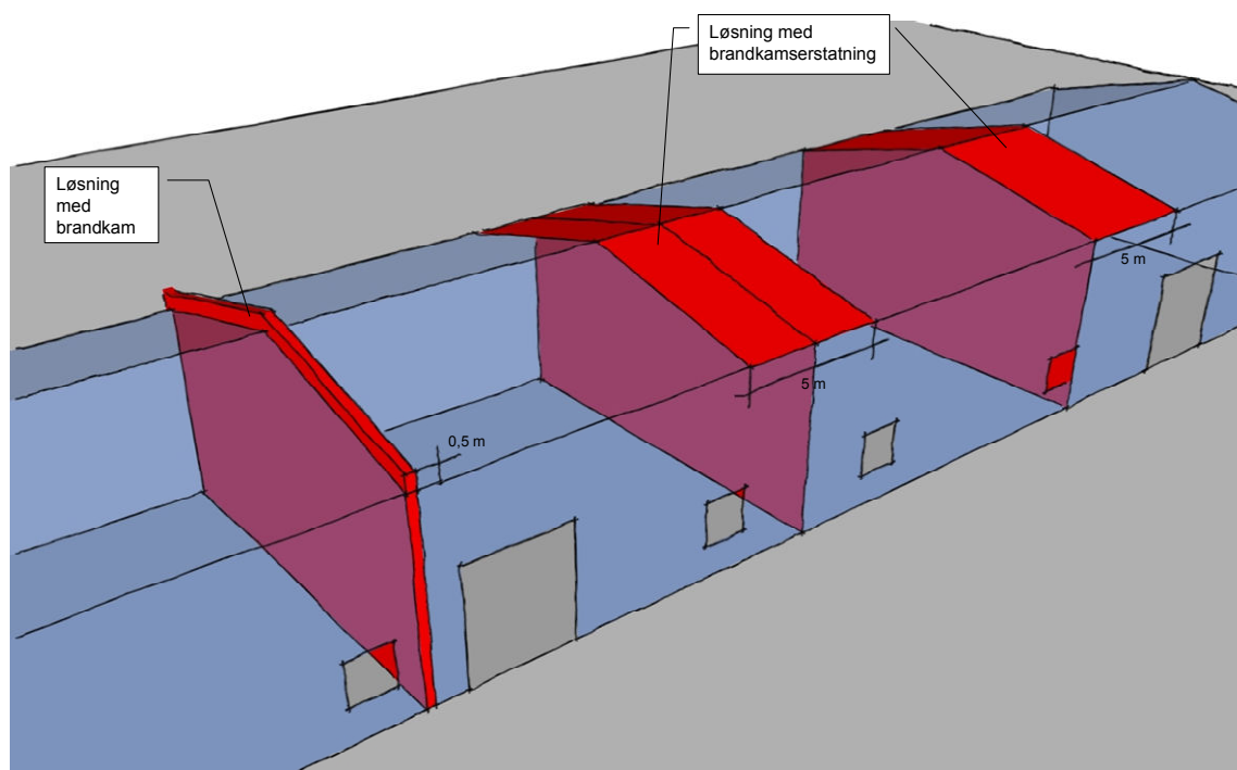
Figur 21: Illustration af løsning med hhv. brandkam, dobbeltsidet og enkeltsidet brandkamserstatning.
