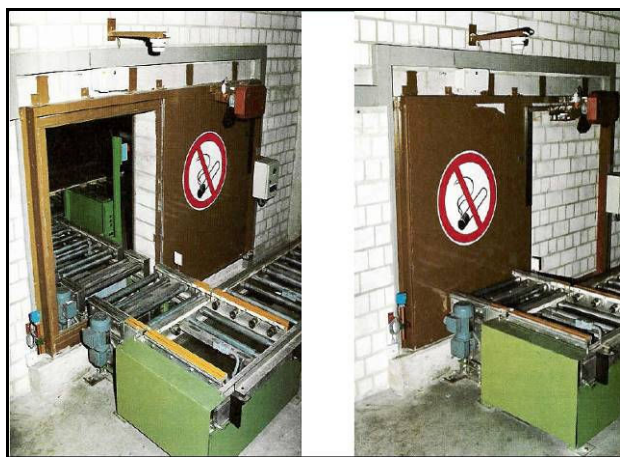
Figur 30: Billede af en transportåbning.
