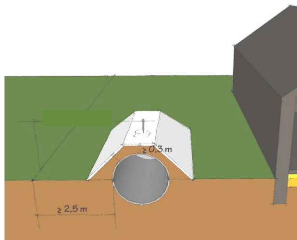
Figur 15: Tank, der er forsynet med en belægning eller lignende, som sikrer, at jordlaget forbliver intakt og dermed bevarer jordlagstykkelsen.
