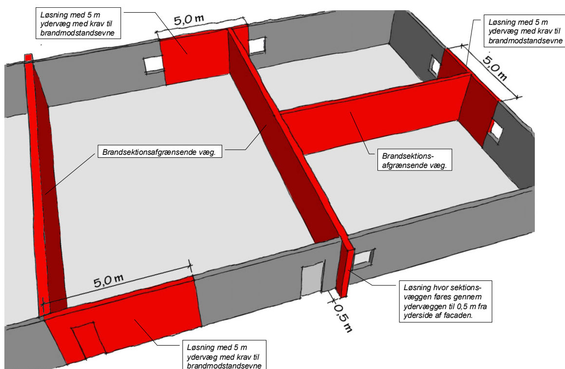
Figur 19: Eksempel på sikring mod brandsmitte (facadesmitte) i ydervæggen.
