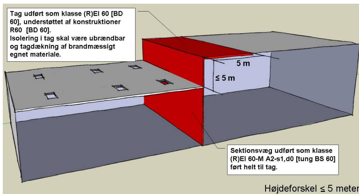
Figur 26: Sikring mod høj-lav brandsmitte, hvor den højere bygnings tag er mindre end eller lig med 5 m over den lavere bygnings tag. Løsning med brandkamserstatning. Der henvises til vejledningens afsnit om brandkamserstatning for udførelse af tagdækning i brandmæssigt egnet materiale.
