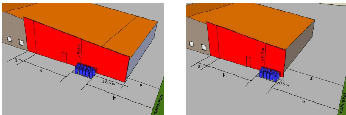
Figur 36: Eksempel på bortfald af den indbyrdes afstand, ved oplag mod bygning, ved etablering af brandsektionsadskillelse inden for den krævede afstand. "Den krævede afstand" svarer til den indbyrdes afstand fundet vha. "sumreglen". I figuren til venstre skal der ikke etableres sikring mod brandsmitte i gavlen, da afstanden overstiger 5 m. I figuren til højre er der vist sikring mod brandsmitte i gavlen, idet brandsektionsadskillelsen er videreført til en afstand af 0,5 m fra bygningens ydervæg. Der er udført en brandkam, idet afstanden fra oplaget til taget er mindre end 5 m.
