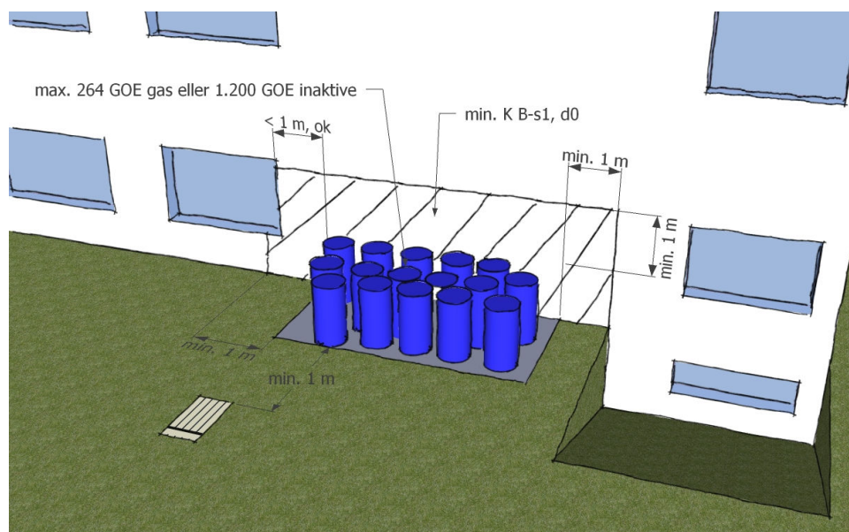
Figur 9: Illustration af afstandforhold, der gør sig gældende, hvis afstandskrav for lagerafsnit i det fri skal bortfalde i forhold til fleretages bygninger, som alene er omfattet af bygningsreglementet.
