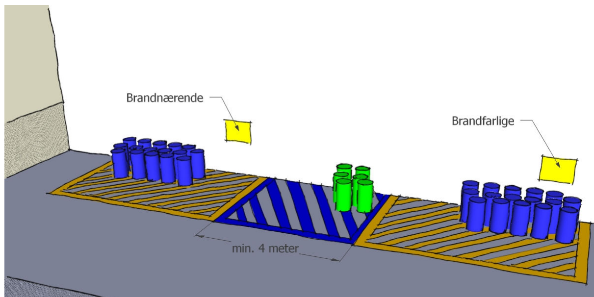
Figur 11: Eksempel på markering på belægning i det fri ved oplag af gasser.
