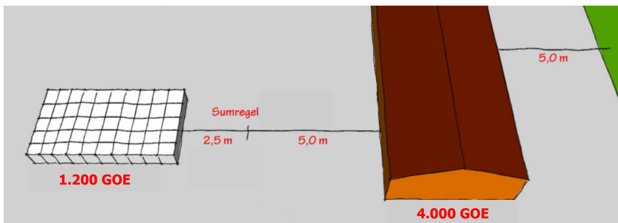
Figur 35: Et eksempel, hvor det indbyrdes afstandskrav er opfyldt.
