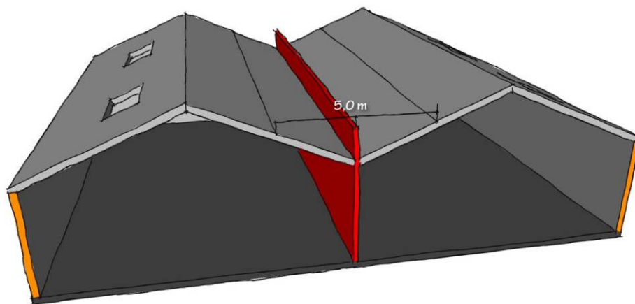
Figur 20: Udførelse af brandkam hvor taghældningen mod brandsektionsvæggen er større end 1:8.
