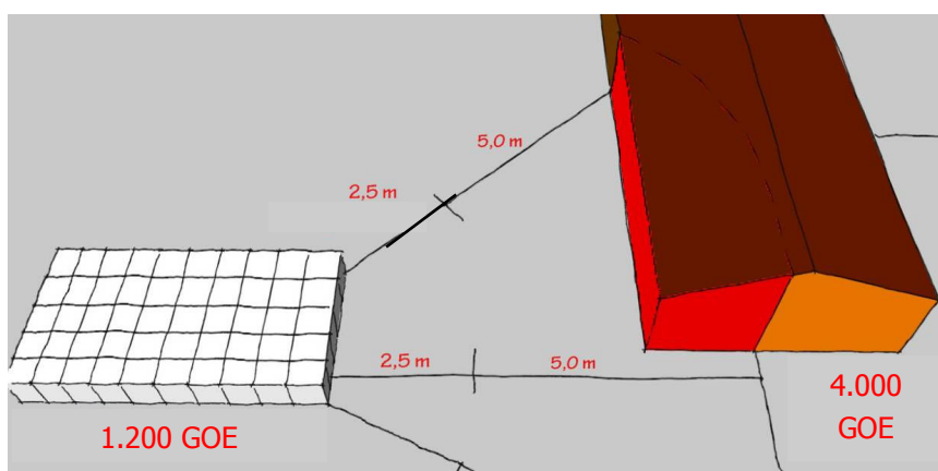
Figur 37: Nedsættelse af den indbyrdes afstand ved oplag mod bygning ved etablering af brandsektionsadskillelse i facaden inden for den krævede afstand (i dette eksempel 7,5 m). Sikring af tag og særlige foranstaltninger mod brandsmitte på gavl-væggen skal kun ske, når den indbyrdes afstand er mindre end 5 m.
