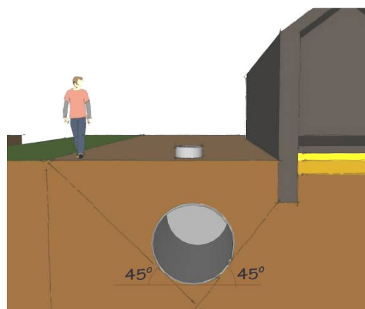
Figur 17: Trykzonen i forhold til bygninger, naboskel og vej kan fastlægges ud fra en 45^\circ vinkel.
