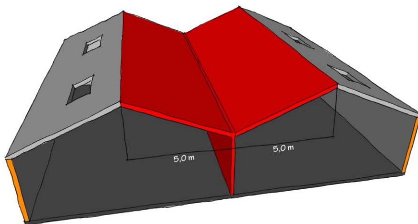
Figur 23: Udførelse af brandkamserstatning hvor taghældningen mod brandsektionsvæggen er større end 1:8. Sikringen skal udføres som mindst EI 60 (ikke bærende, adskillende BD-bygningsdel 60).
