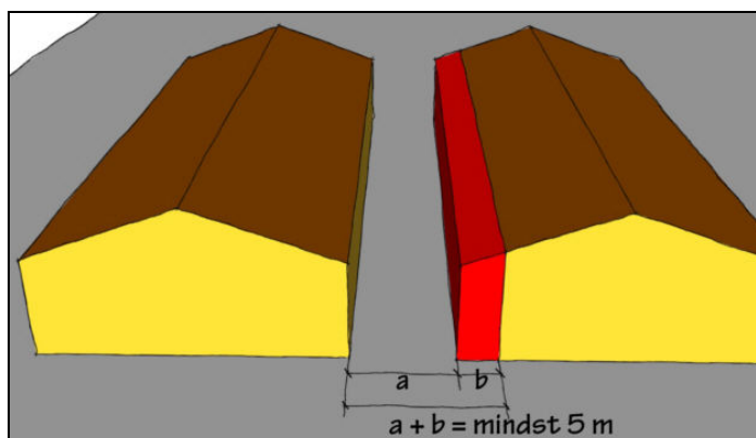
Figur 38: Den krævede indbyrdes afstand er ikke opfyldt mellem to bygninger. Der skal derfor etableres brandsektionsadskillelse, og i en afstand af mindst 5 m skal der i dette eksempel endvidere ske sikring af tag og ydervæg.
