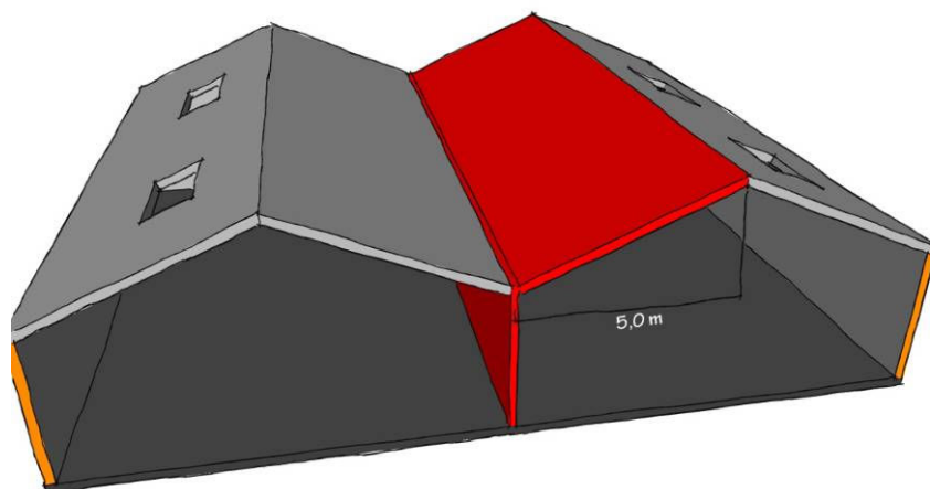
Figur 22: Udførelse af brandkamserstatning hvor taghældningen mod brandsektionsvæggen er større end 1:8. Sikringen skal udføres som mindst REI 60 (bærende, adskillende BD-bygningsdel 60).
