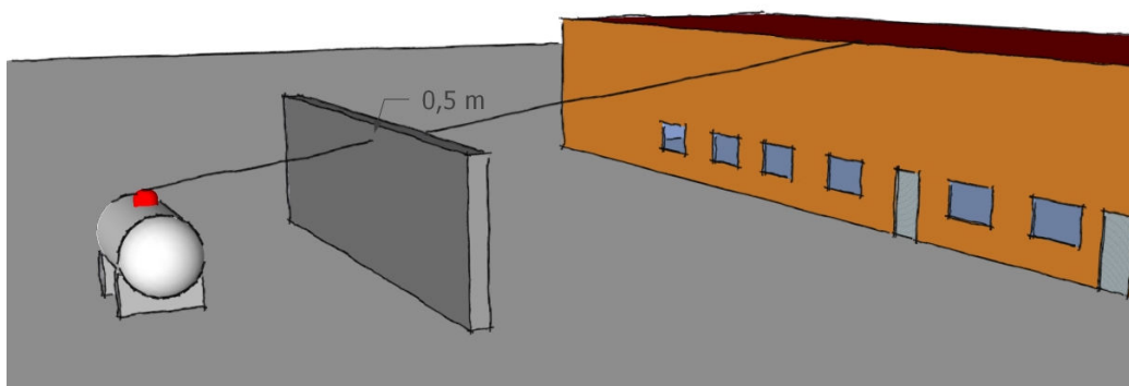
Figur 8: Højde på flammeskærm, 0,5 m højere end sigtelinie.
