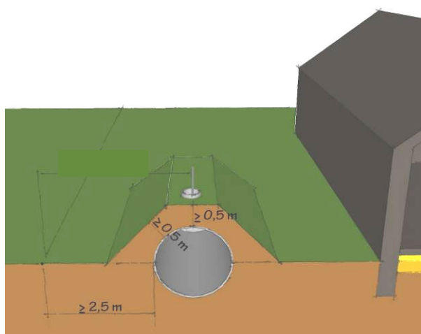
Figur 14: Tank, der er jorddækket med mindst 0,5 m jord.
