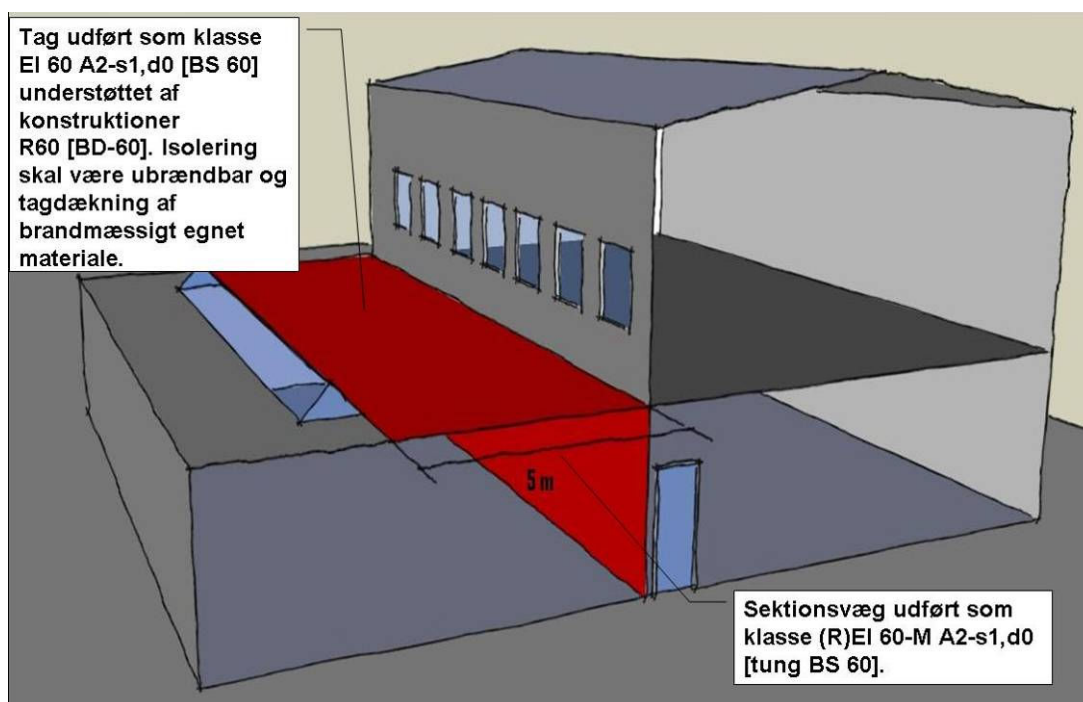
Figur 28: Sikring mod høj-lav brandsmitte, hvor sikringen er udført på den lavere brandsektions tag. Der henvises til vejledningens afsnit om brandkamserstatning for udførelse af tagdækning i brandmæssigt egnet materiale.
