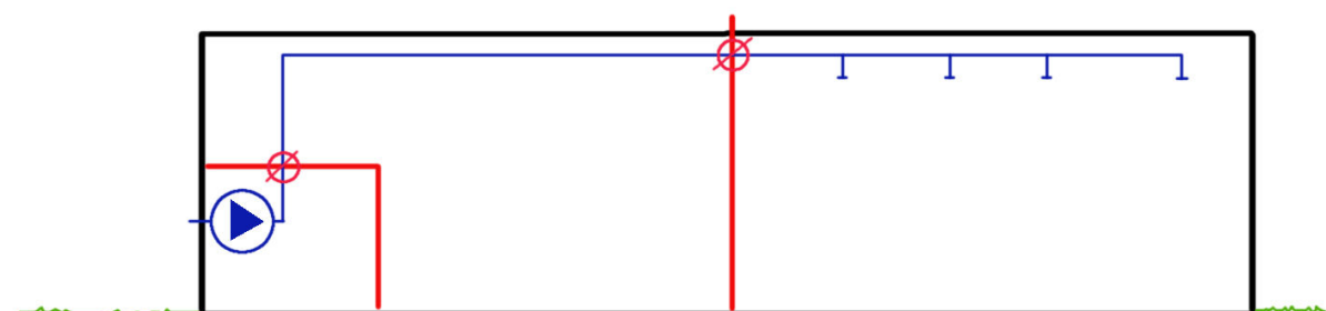
Figur 18: Eksempel på et ventilationsanlæg, der betjener ét lagerafsnit med oplag af brandfarlige gasser (må kun betjene ét lagerafsnit). Kanal gennemføringen mellem brandsektionerne og mellem ventilationsrummet og brandsektion er sikret med et brand- og røgspjæld (BRS-spjæld). Kanalerne er udført af mindst materiale klasse A2-s1,d0 af metal med et smeltepunkt på mindst 850 °C.
