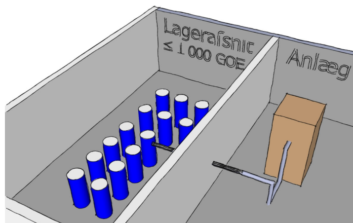
Figur 12: Anlæg med lagerafsnit i bygning. Højest 1.000 gasoplagsenheder.
