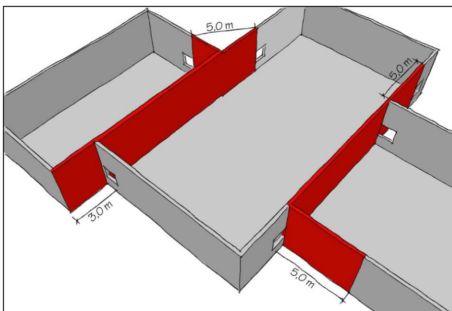
Figur 24: Eksempler på sikring mod vinkelsmitte i ydervægge.
