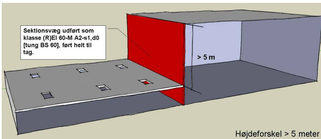
Figur 27: Sikring mod høj-lav brandsmitte, hvor den højere bygnings tag er større end 5 m over den lavere bygnings tag. Ingen krav om brandkam eller brandkamserstatning.
