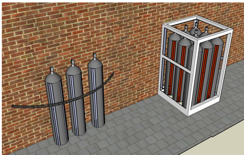
Figur 10: Illustration af sikring mod væltning.
